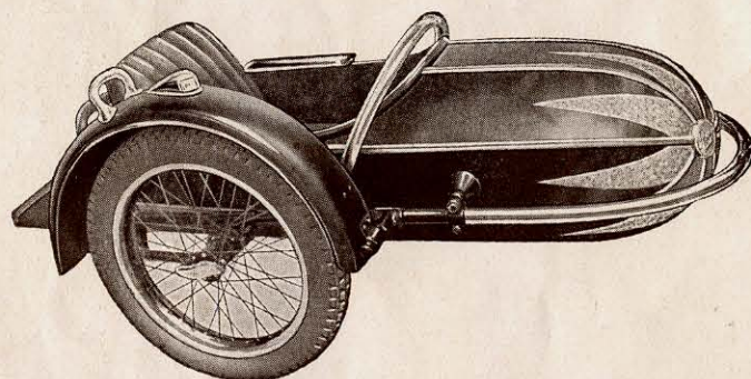
Sport-Seitenwagen Nr. 36 aus glattem Aluminiumblech, emailliert mit touchiertem Stern, oder Sport-Seitenwagen Nr. 37 (Form wie Nr. 36) aus glattem Stahlblech, emal- liert, Farbe nach Wunsch RM. 220.—
