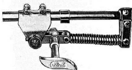
Steib Schwingachse, ge- lagert auf 2 doppelreihigen Präzisions-Kugellagern
